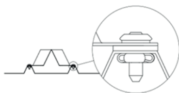
Fixação com 12 rebites 7,7 Bulb-Tite®
